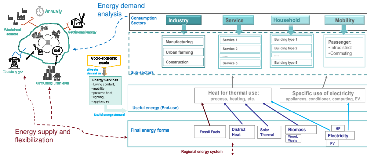
Abbildung 2: MAPED-Konzept zur Aufschlüsselung des Energiebedarfs des Stadtteils nach Brennstoffen und Verbrauchssektoren sowie zur geplanten Energieversorgung und zum Energieaustausch mit dem Nachbarschaftsenergiesystem ©AIT
